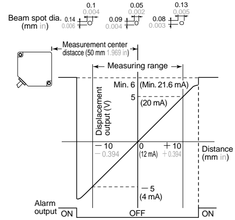
ANR1151 ANR1251
